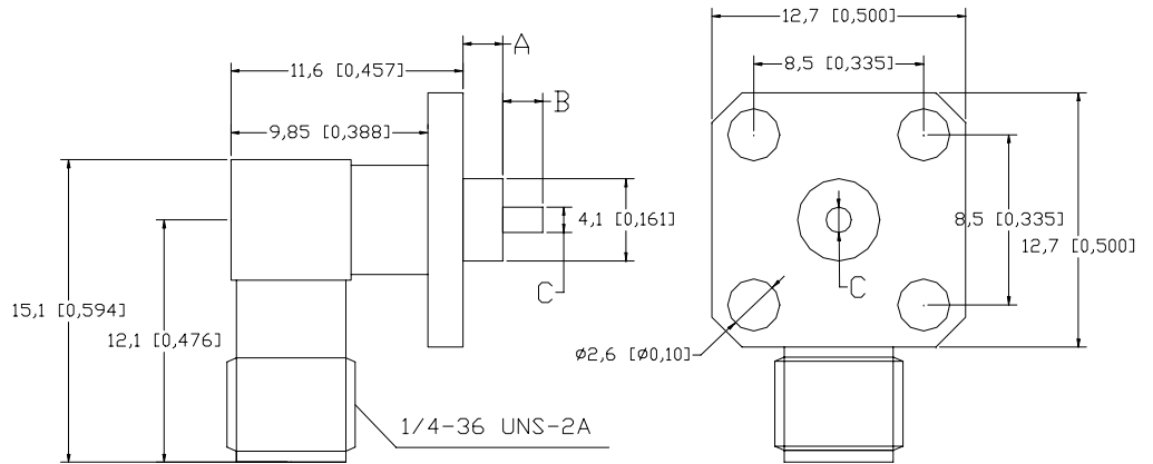
Unit : mm[inch]
